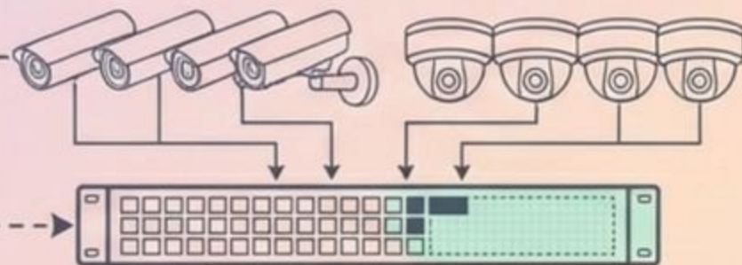
NVR B 偵測到異常，立即啟用其 156 CH 的保留容量。同時管理原有的 100 台 + 接管自 NVR A 的 100 台攝影機，維持 200 台攝影機穩定錄影。
